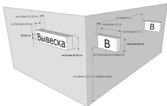
Размеры вывески
